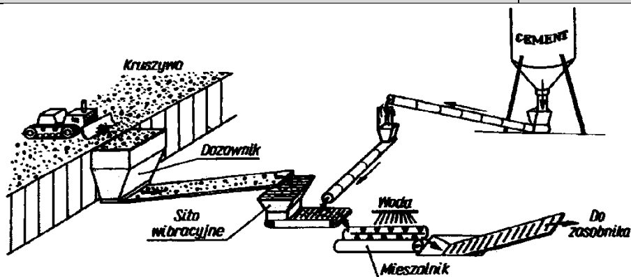
Rys. 7. Schemat technologiczny wytwarzania mieszanki kruszywa związanej cementem w mieszarce o działaniu ciągłym (wg: S. Rolla, M. Rolla i W. Żarnoż – Budowa dróg cz. 1. Wyd. Szkolne i Pedagogiczne, 1993)
