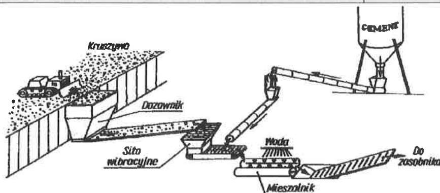
Rys. 7. Schemat technologiczny wytwarzania mieszanki kruszywa związanej cementem w mieszarce o działaniu ciągłym (wg: S. Rolla, M. Rolla i W. Żarnoch – Budowa dróg cz. 1. Wyd. Szkolne i Pedagogiczne, 1993)
