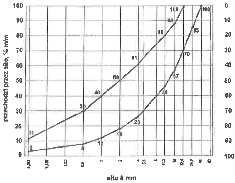
Rys. 1. Krzywe graniczne uziarnienia mieszanki mineralnej 0/31,5 mm
