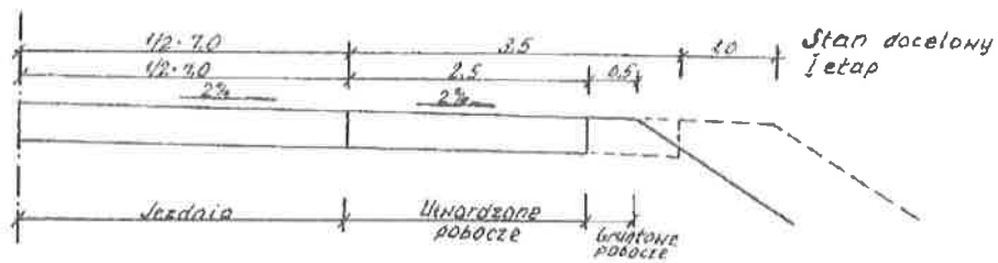
Rys. 3. Konstrukcja nawierzchni utwardzonego pobocza
