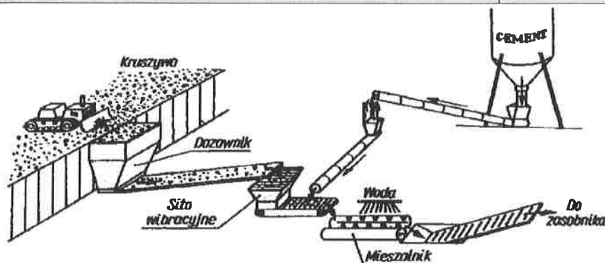
Rys. 7. Schemat technologiczny wytwarzania mieszanki kruszywa związanej cementem w mieszarce o działaniu ciągłym (wg: S. Rolla, M. Rolla i W. Żarnoch – Budowa dróg cz. 1. Wyd. Szkolne i Pedagogiczne, 1993)
